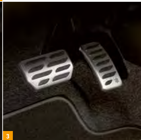
3 | Set pedaliera Sportiva in alluminio per lato SX e DX per cambio manuale (no foto) codice 990E0-61M93-000 per cambio automatico codice 990E0-61M93-001
